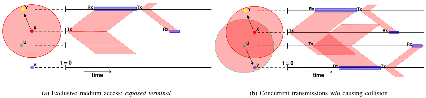
Fig. 3. Spatial Reuse
