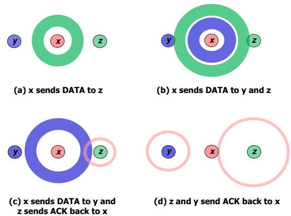
Fig. 2. Temporal Reuse
